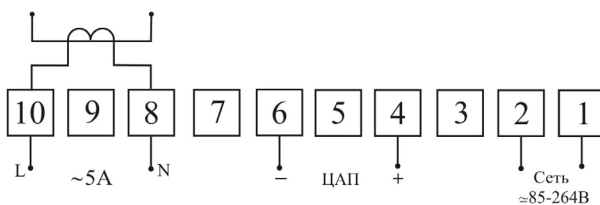
Рис. 4 – Клеммы подключения P94-A-1-0.5-I420
