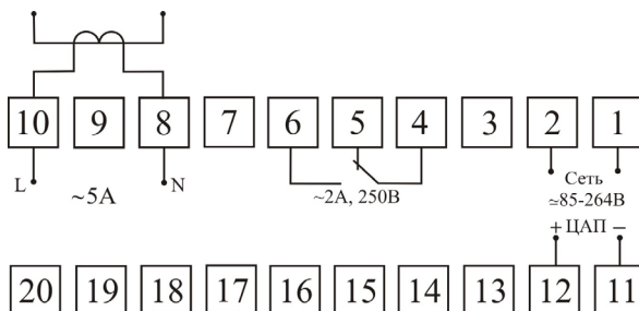
Рис. 6 – Клеммы подключения P94-A-1-0.5-K-I420
